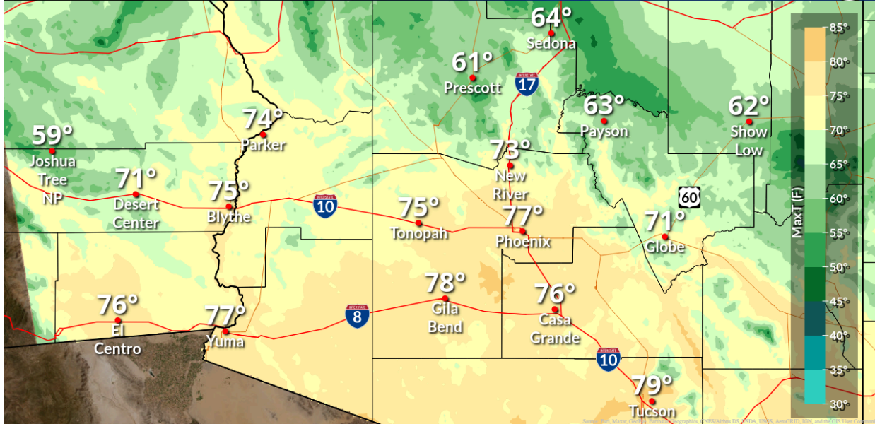
MaxT_Day6.png
