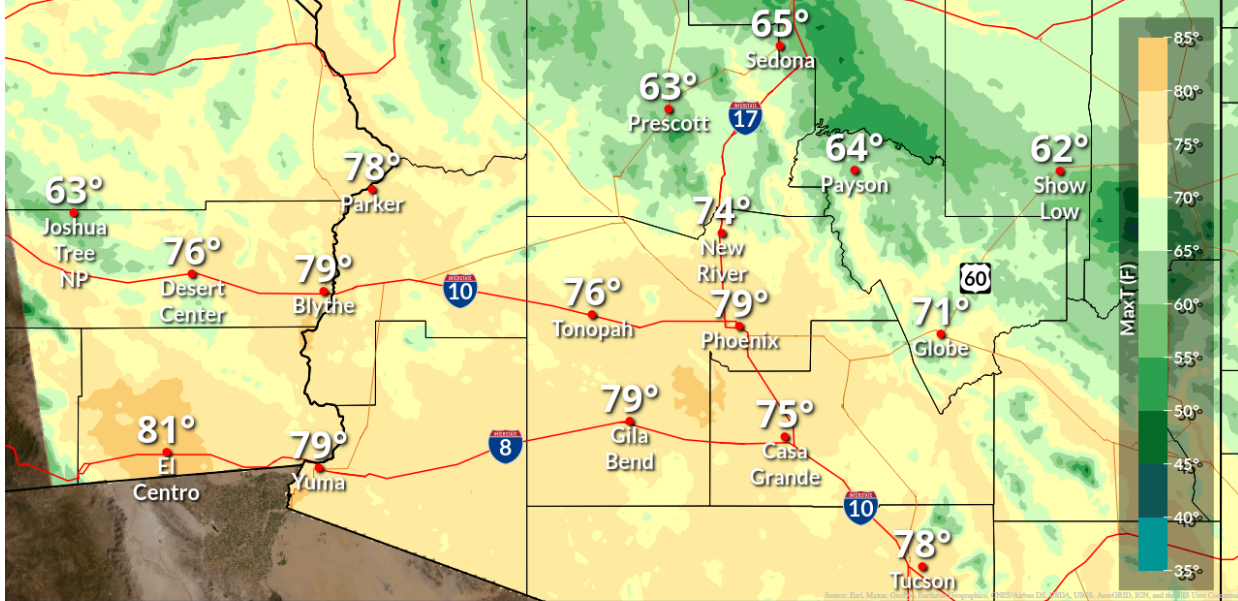
MaxT_Day3.png
